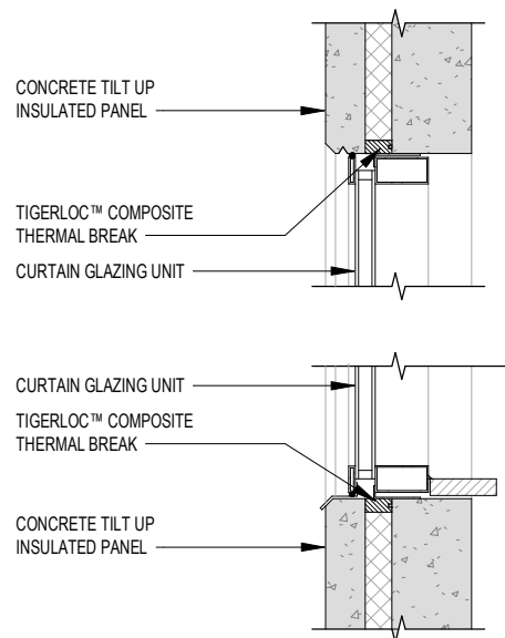
CURTAINWALL
