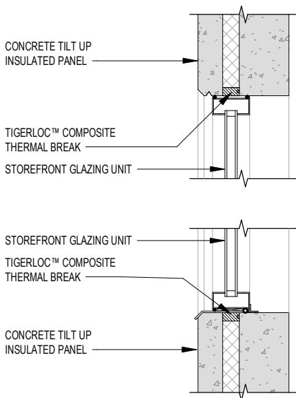
STOREFRONT
