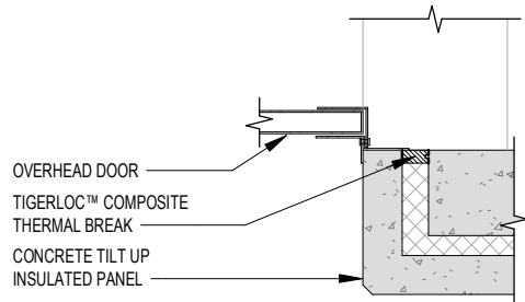
OVERHEAD DOOR
